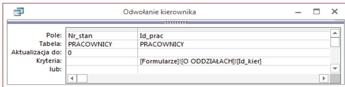
Rys. 2. Kwerenda aktualizująca Odwołanie kierownika – siatka projektowa
